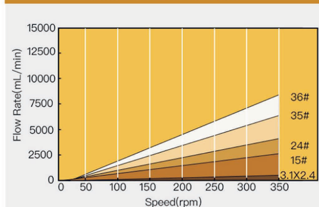
Flow Rate(0.1-350rpm)
